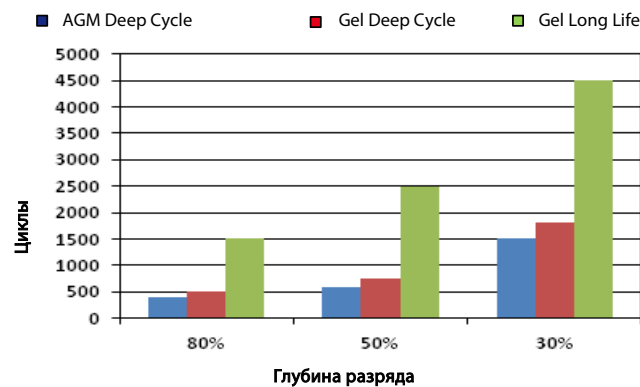
Рис. 2: Эксплуатационные циклы
