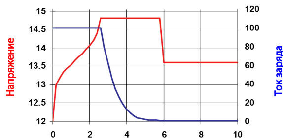
Рис. 3: Трехступенчатая кривая заряда
