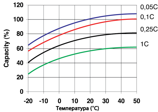
Рис. 1: Эффект температуры на емкость
