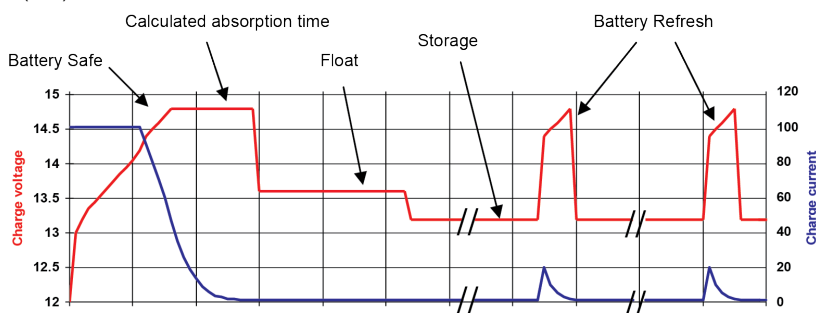
Рис. 4: Четырехступенчатая адаптивная кривая заряда
